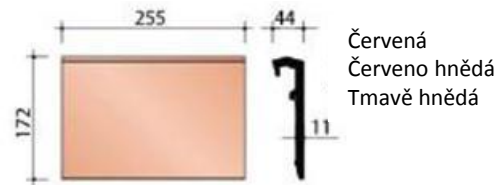
Koncová keramická tvarovka
