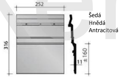
Koncová keramická tvarovka
