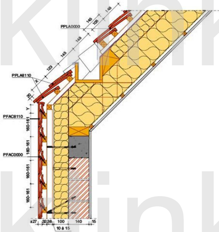
Koncová keramická tvarovka
